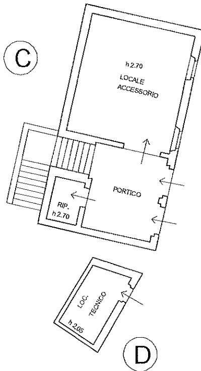
PIANO S1 (SEMINTERRATO)
