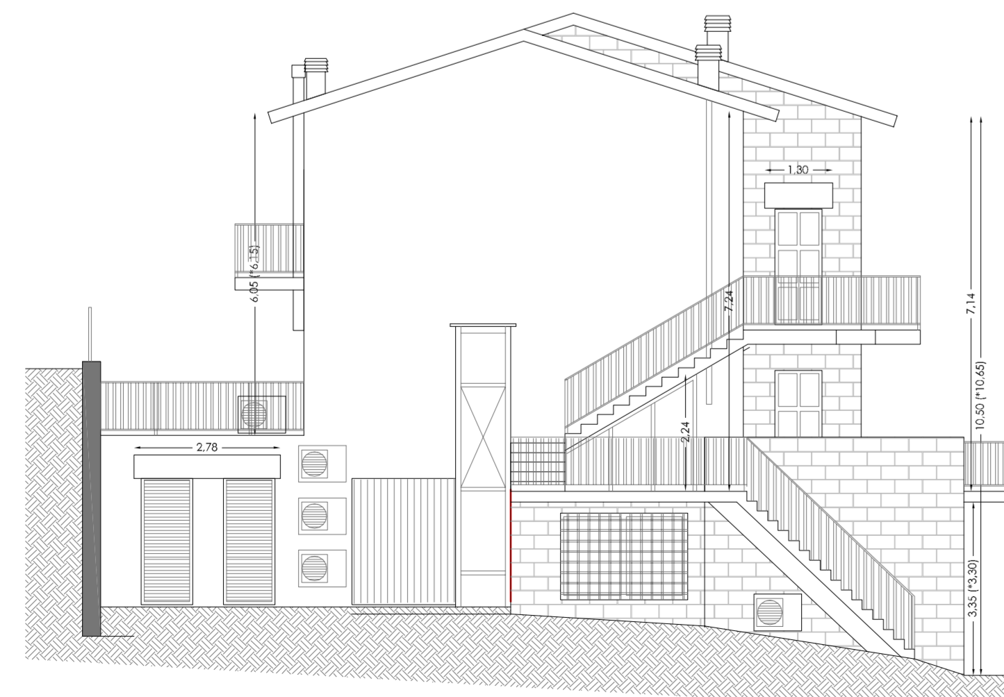
PROSPETTO EST
