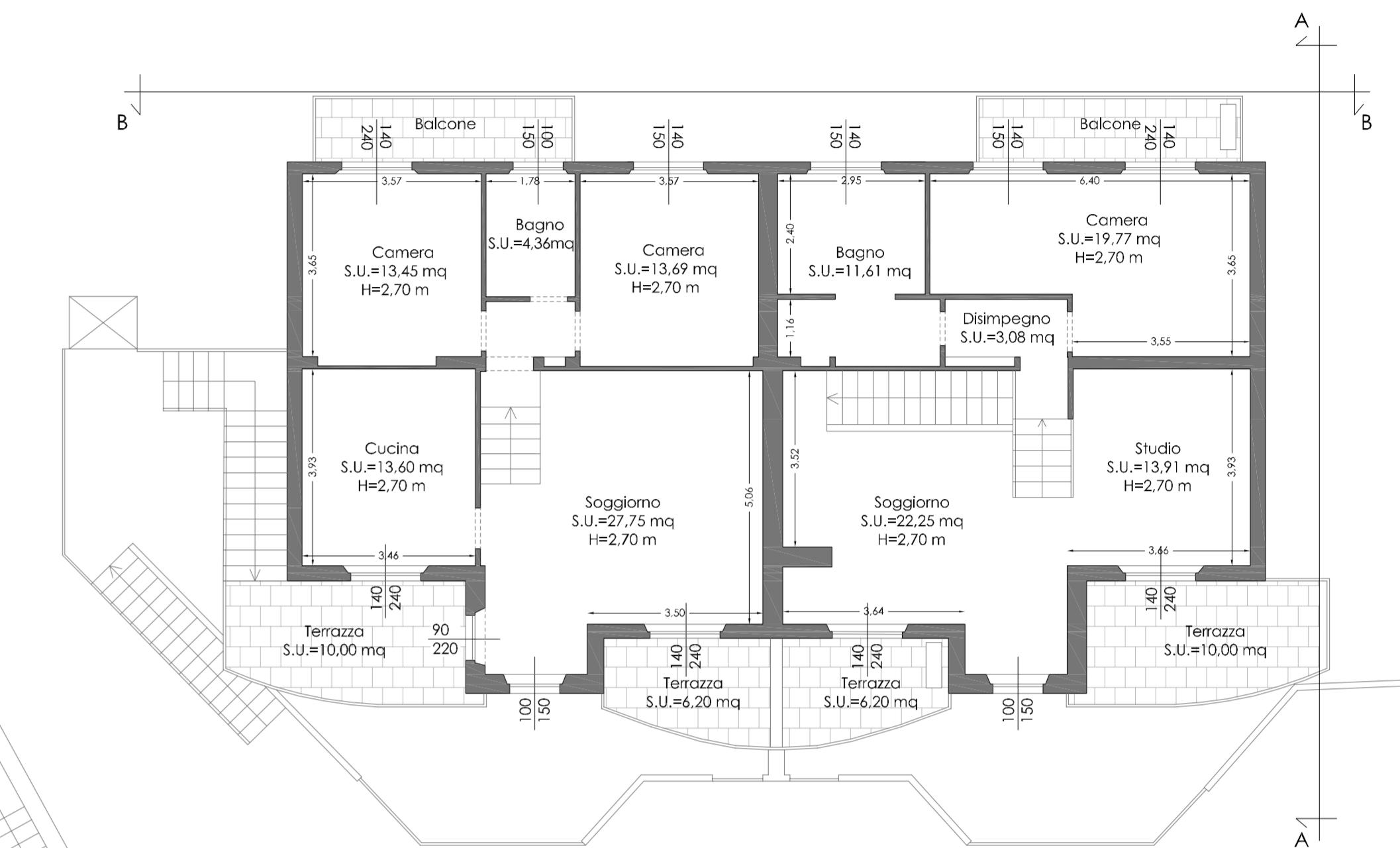
PIANO PRIMO
