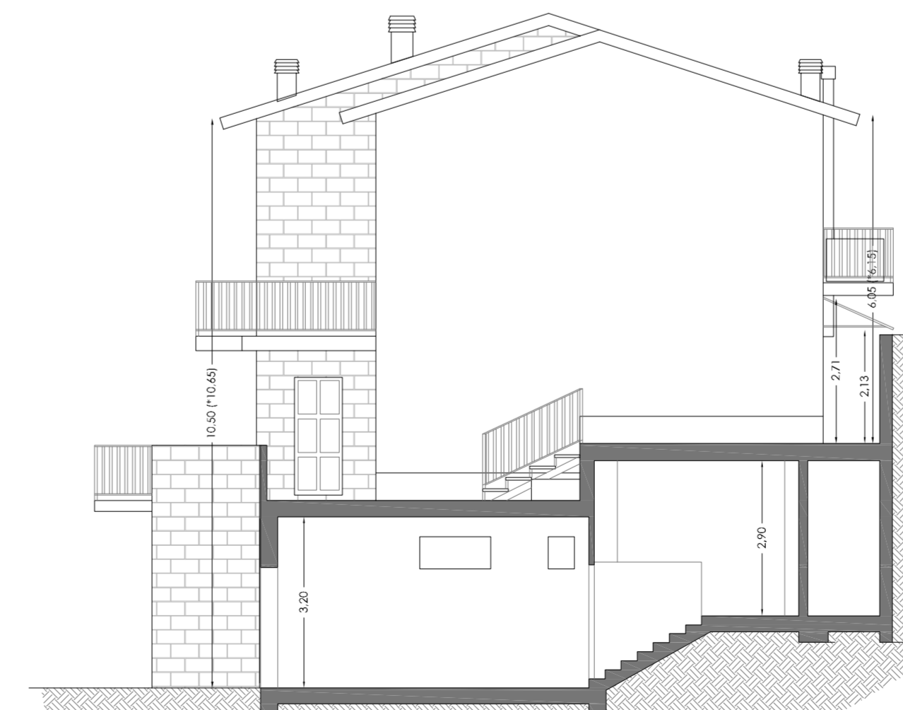
PROSPETTO OVEST (sezione A-A)
